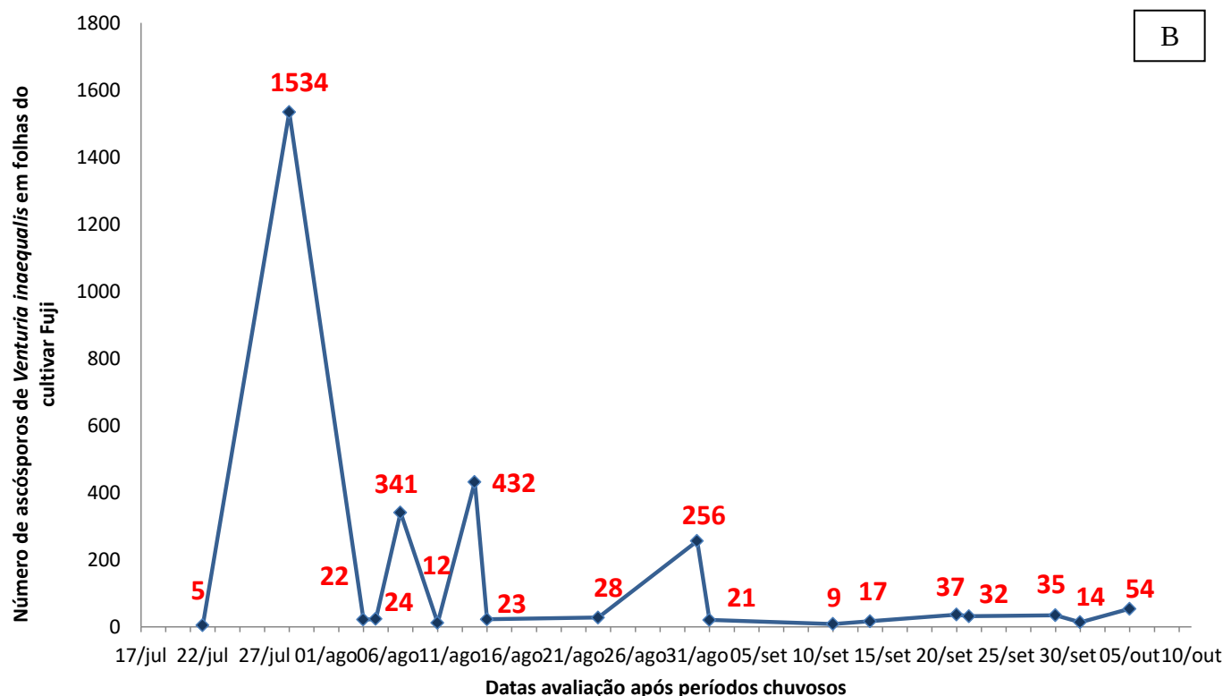
Figura 1 – Número de ascósporos de Venturia inaequalis ejetados ao longo do tempo e capturados em armadilhas contendo folhas dos cultivares Gala (A) e Fuji (B) mantidos na Estação Experimental de São Joaquim da Epagri.
