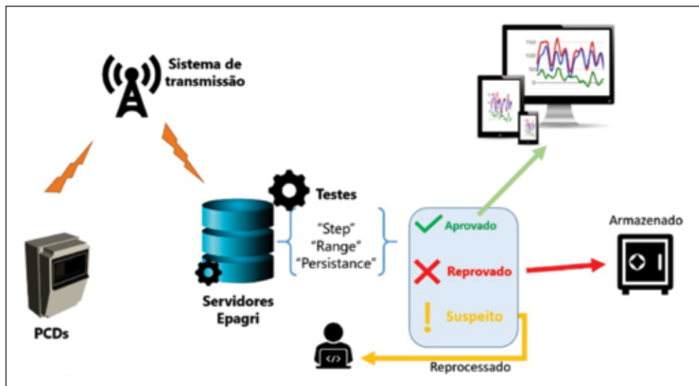
Figura 3. Esquema de funcionamento do sistema de qualificação de dados ambientais da Epagri/Ciram
