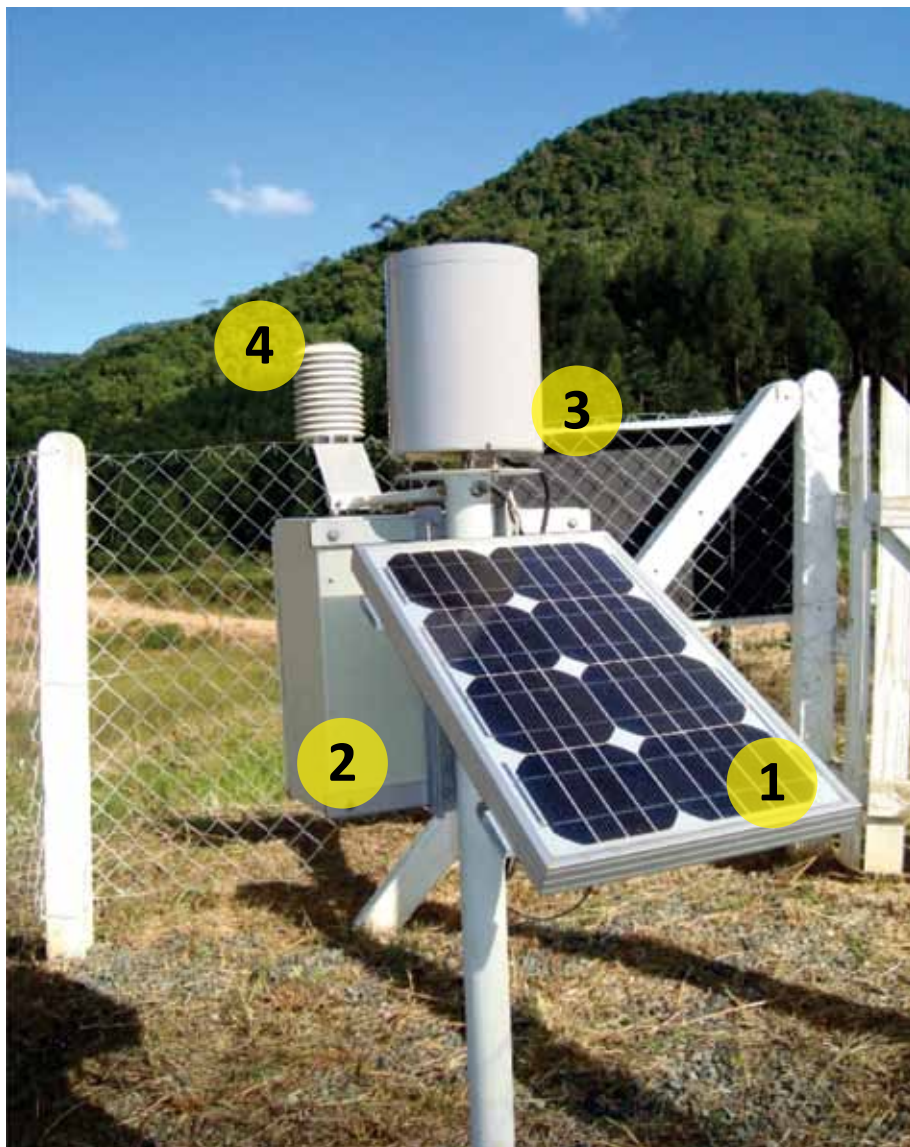
Figura 1. Exemplo de PCD agrometeorológica Foto: Éverton Blainski
